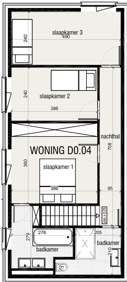
1STE VERDIEPING
