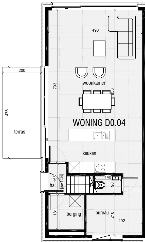
GELIJKVLOERS
